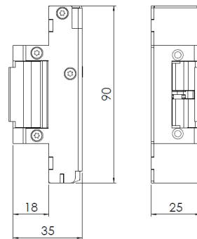
Måttskiss STEP 98 Preload.
